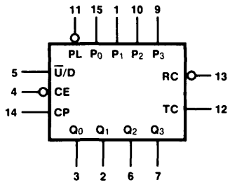
D130 54/74190, 74LS190 54/74191, 74LS191
