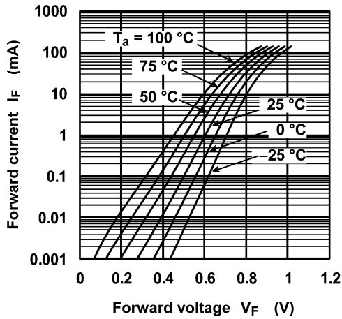
Fig. 7.1 I_F - V_F
