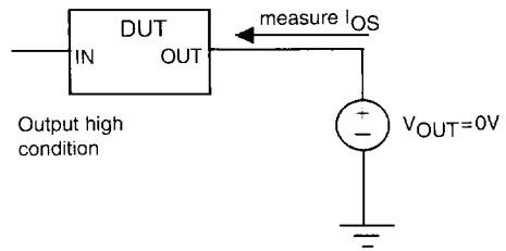
FIG. 5 I_{OS} Test
