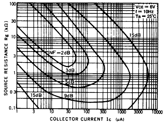
Fig.16 雑音特性 (II)
