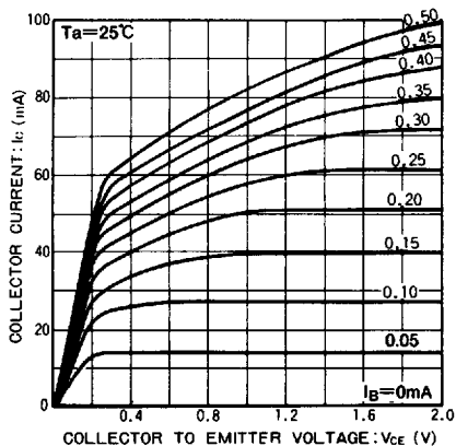
Fig.3 エミッタ接地出力静特性 (I)
