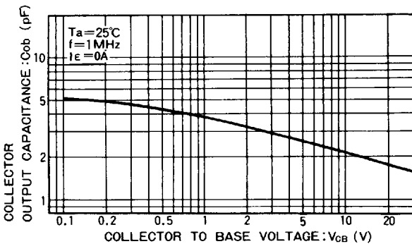
Fig.11 コレクタ出力容量—コレクタ・ベース電圧特性
