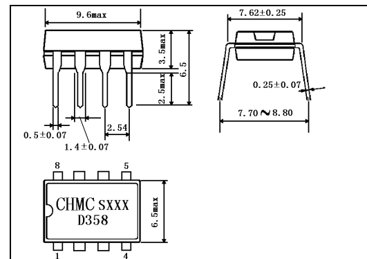
DIP-8
