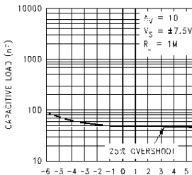
V_{O_U-} (V) DS011713-89
