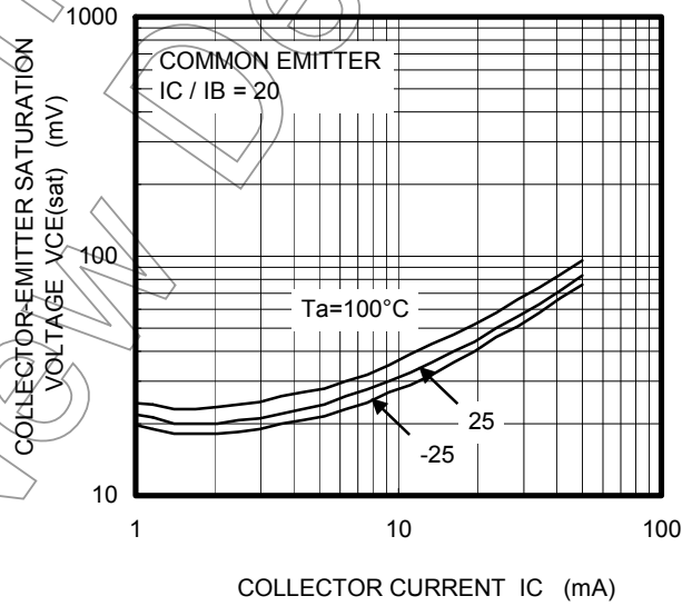
VCE(sat) - IC
