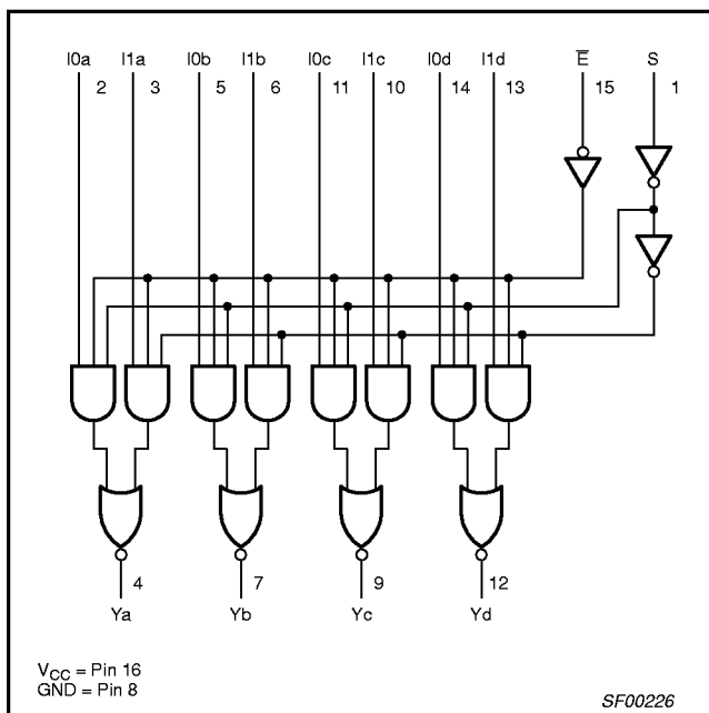
74F158A
