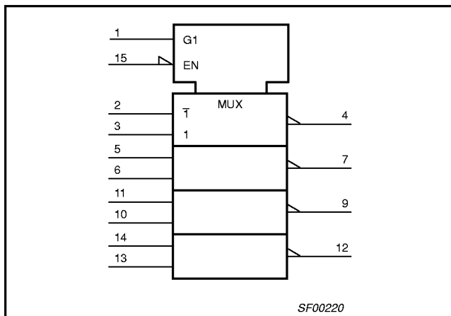
74F158A
