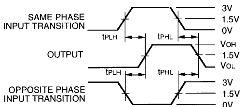
2549 drw 08
