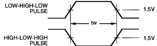
2549 drw 07
