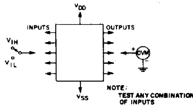
Fig. 13 - Input-voltage test circuit.
