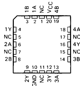
SN54ALS1003A . . . FK PACKAGE
