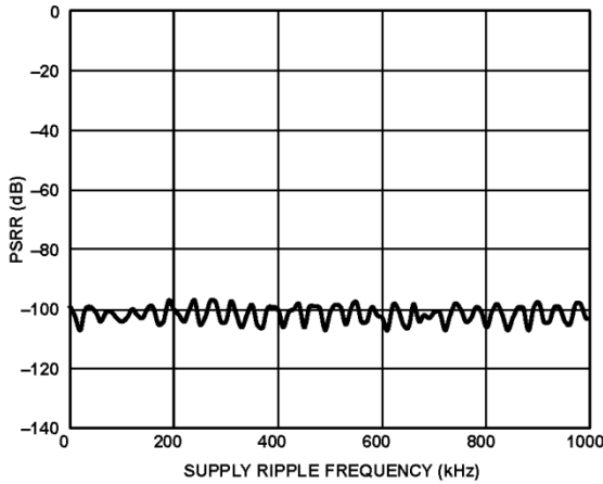
图7. 电源电压抑制比 (PSRR) 与电源纹波频率的关系
