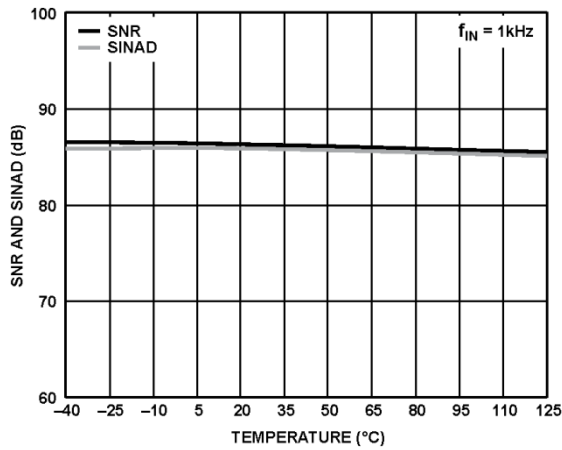
图14. SNR和SINAD与温度的关系
