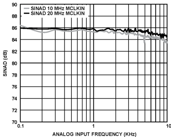
图9. SINAD与模拟输入频率的关系
