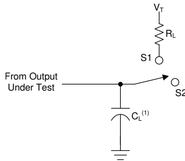
图 7-1. Load Circuit
