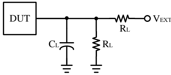
图3 外围负载
