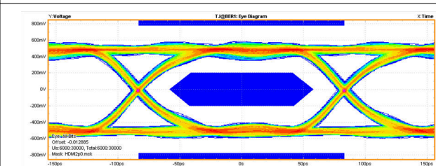
图 8-7. 6-Gbps HDMI 2.0 (TP1) Eye Diagram TPD1E05U06
