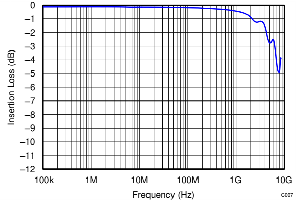
图 6-8. TPD1E05U06 Insertion Loss
