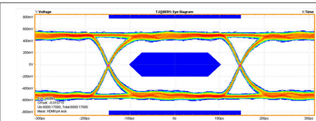
图 8-3. 3.4-Gbps HDMI 1.4 TP1 Eye Diagram TPD1E05U06
