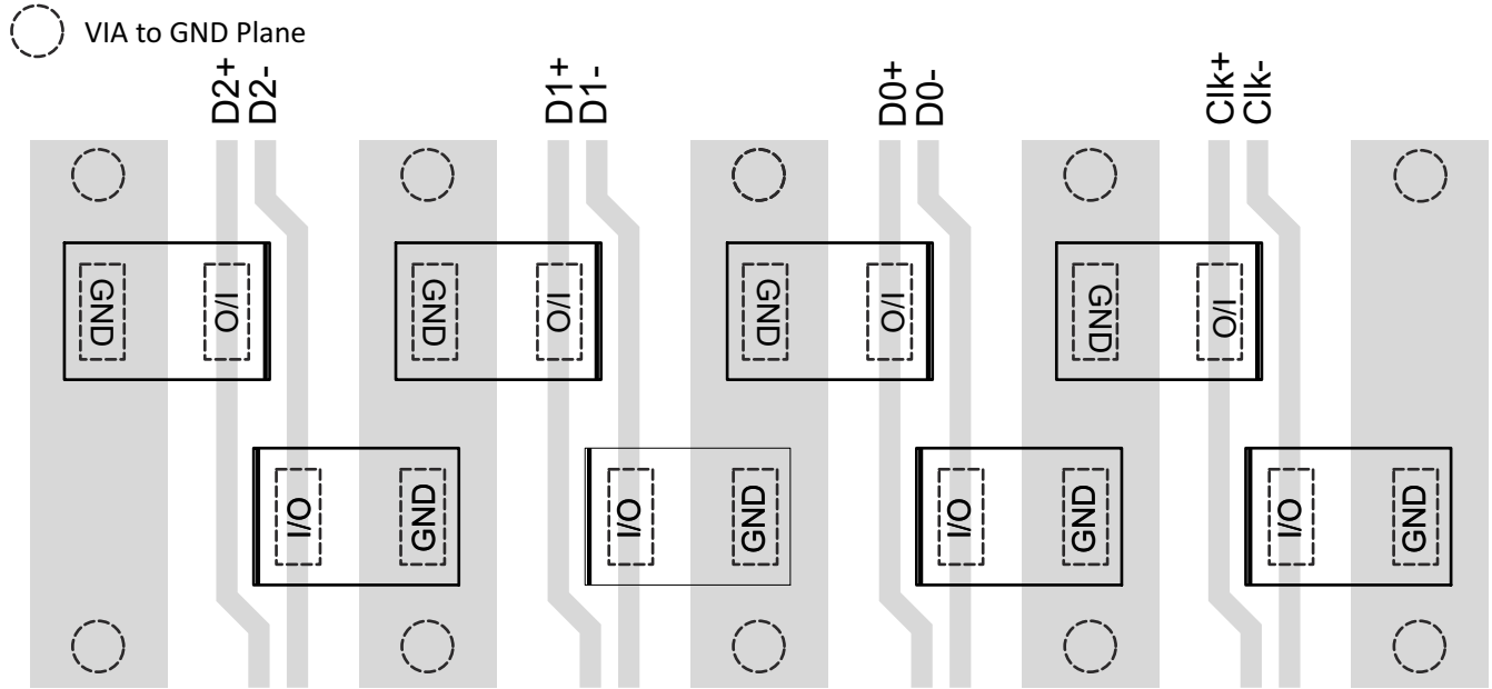
图 10-2. TPD1E05U06 Layout
