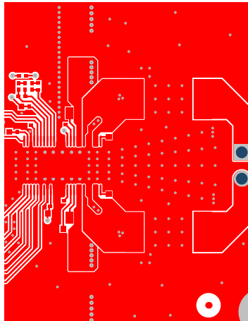
图 74. Layout Example (Mono) - Top Layer
