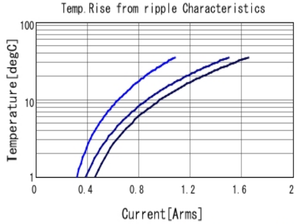
GRM188R61E104KA01 Temp. rise ■ 400kHz ■ 800kHz ■ 1MHz
