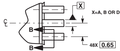
VIEW Y
